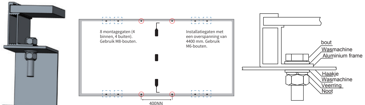
Afbeelding 4 Illustratie van montagegaten voor enkelzijdige componenten
