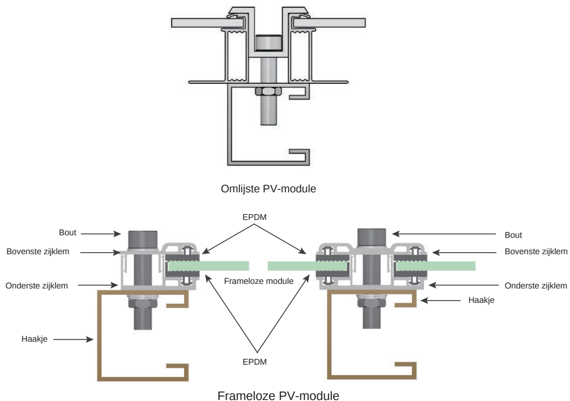
Afbeelding 8 Kleminstallatie van bifaciale module
