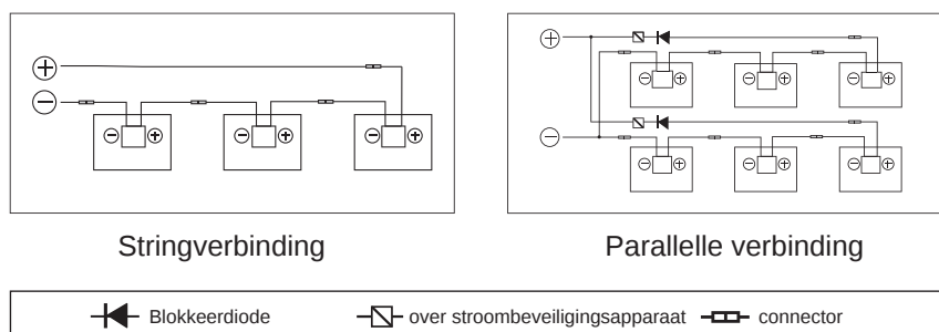
Afbeelding 10 Schakelschema serie-aansluiting en parallelle aansluiting
