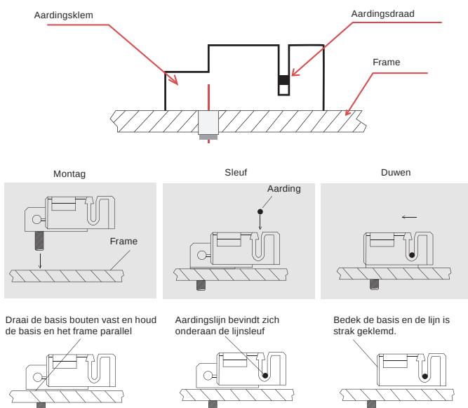
Afbeelding 11 Aardingsmethode voor klem
