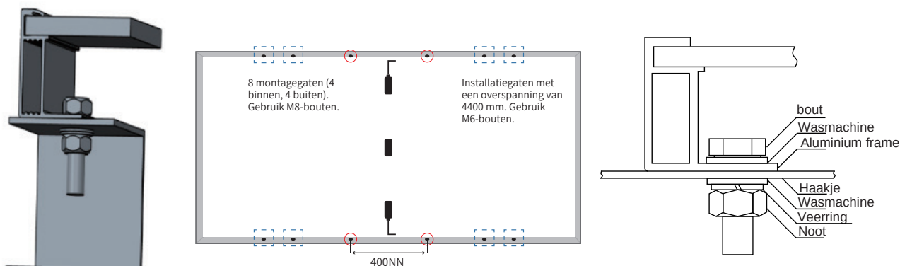
Afbeelding 4 Illustratie van montagegaten voor enkelzijdige componenten
