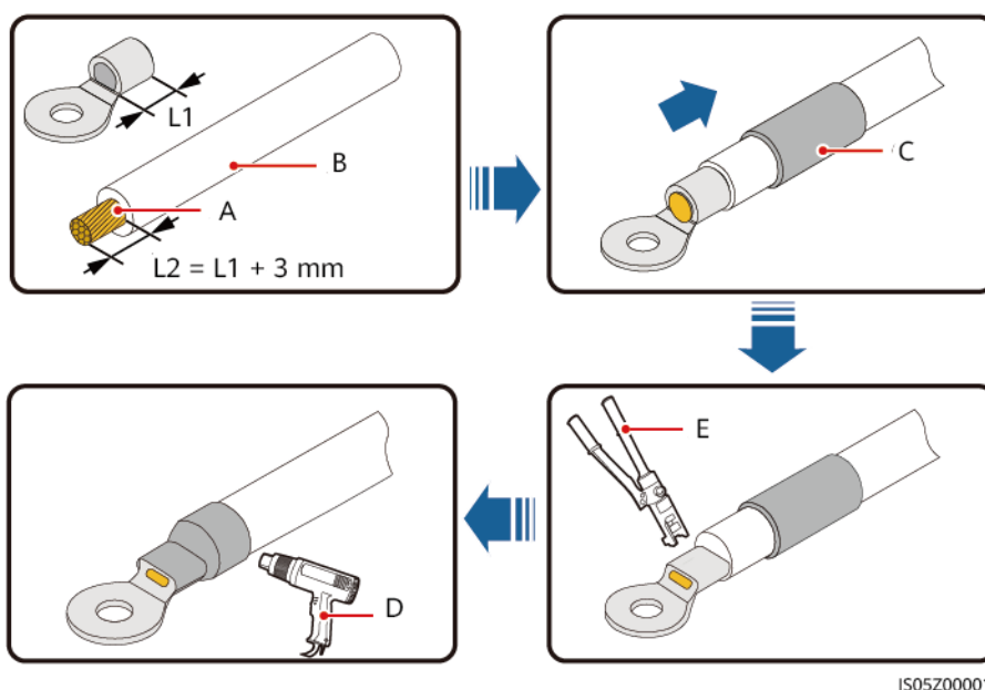
Rysunek 6-9 Zaciśkanie końcówki oczkowej
