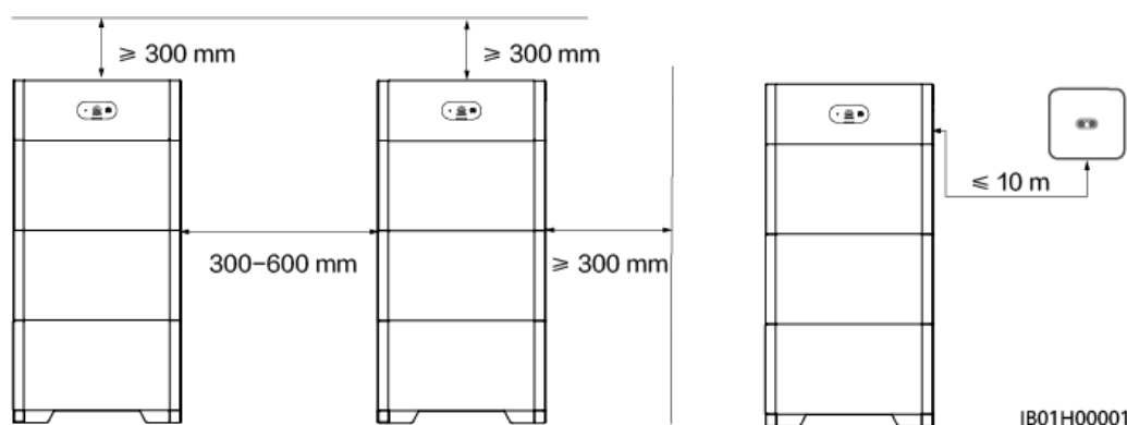
Rysunek 5-1 Miejsce do montażu
