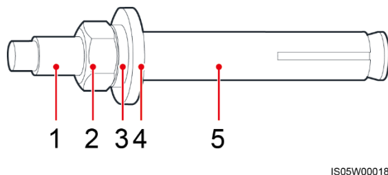
Rysunek 5-3 Schemat struktury kotwy rozporowej M6
