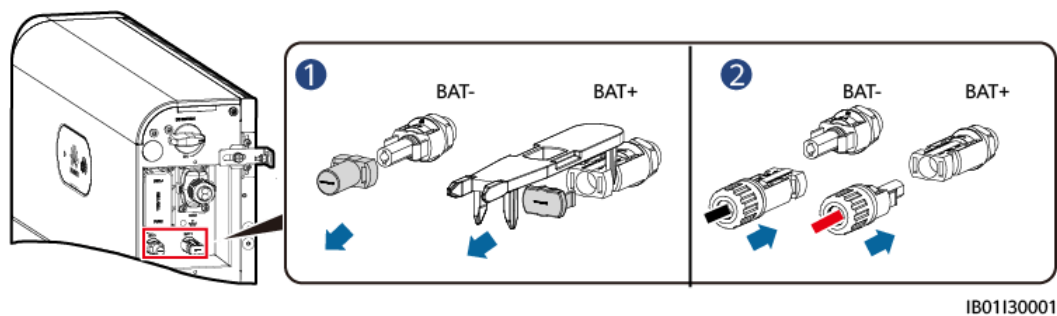
Rysunek 6-12 Podłączanie przewodów baterii
