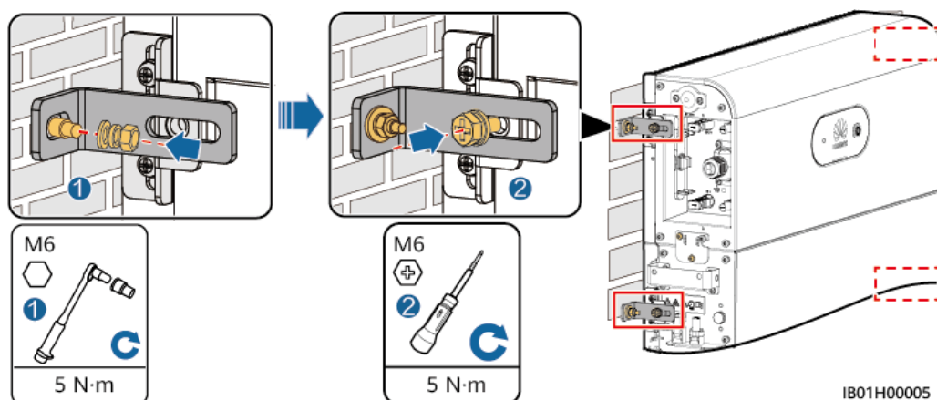
Rysunek 5-6 Mocowanie modułu sterowania zasilaniem
