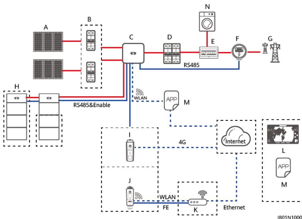
Rysunek 4-1 Schemat połączenia sieciowego systemu magazynowania energii z przyłączem do sieci (kreskowane pola oznaczają komponenty opcjonalne)
