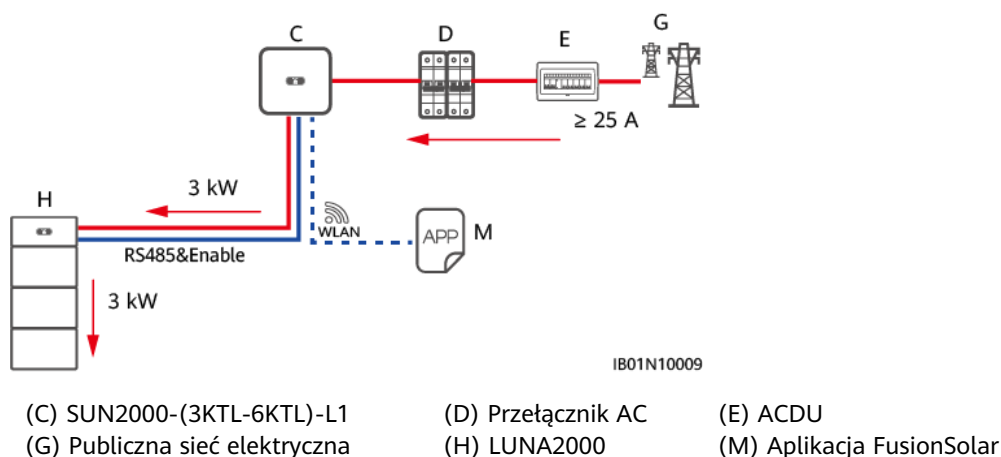
Rysunek 8-2 Schemat połączeń dla scenariusza zasilania pojedynczej fazy
