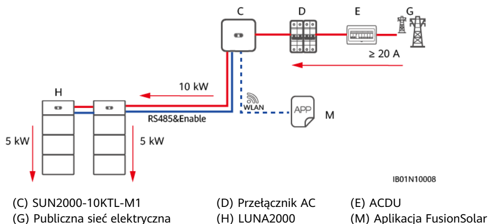
Rysunek 8-1 Schemat połączeń dla scenariusza zasilania trójfazowego
