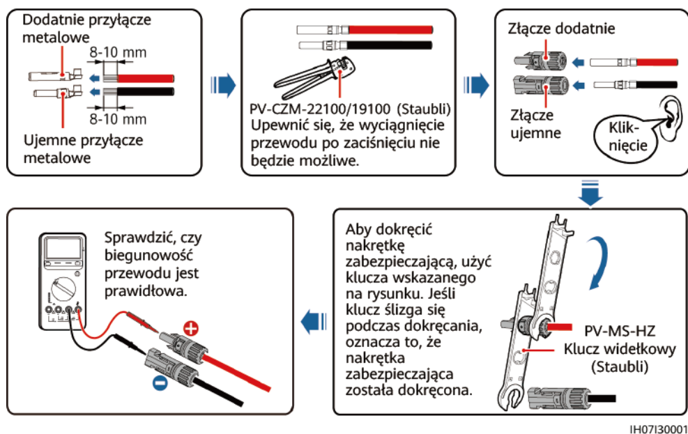
Rysunek 6-11 Montaż złączy prądu stałego
