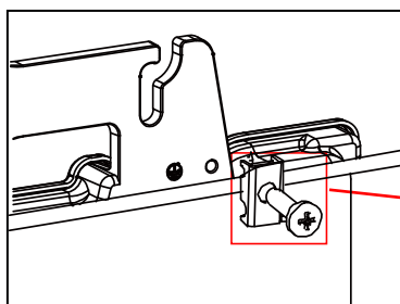
Maadoituskorvake
