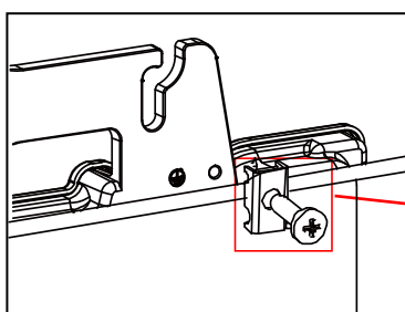
końcówka uziemiająca
